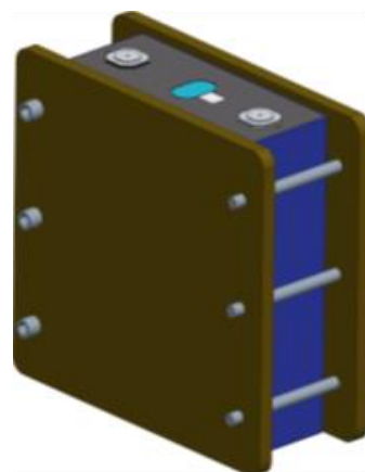
Fig. 4 Diagram of cell with clamp 图 4 电池上夹具图
